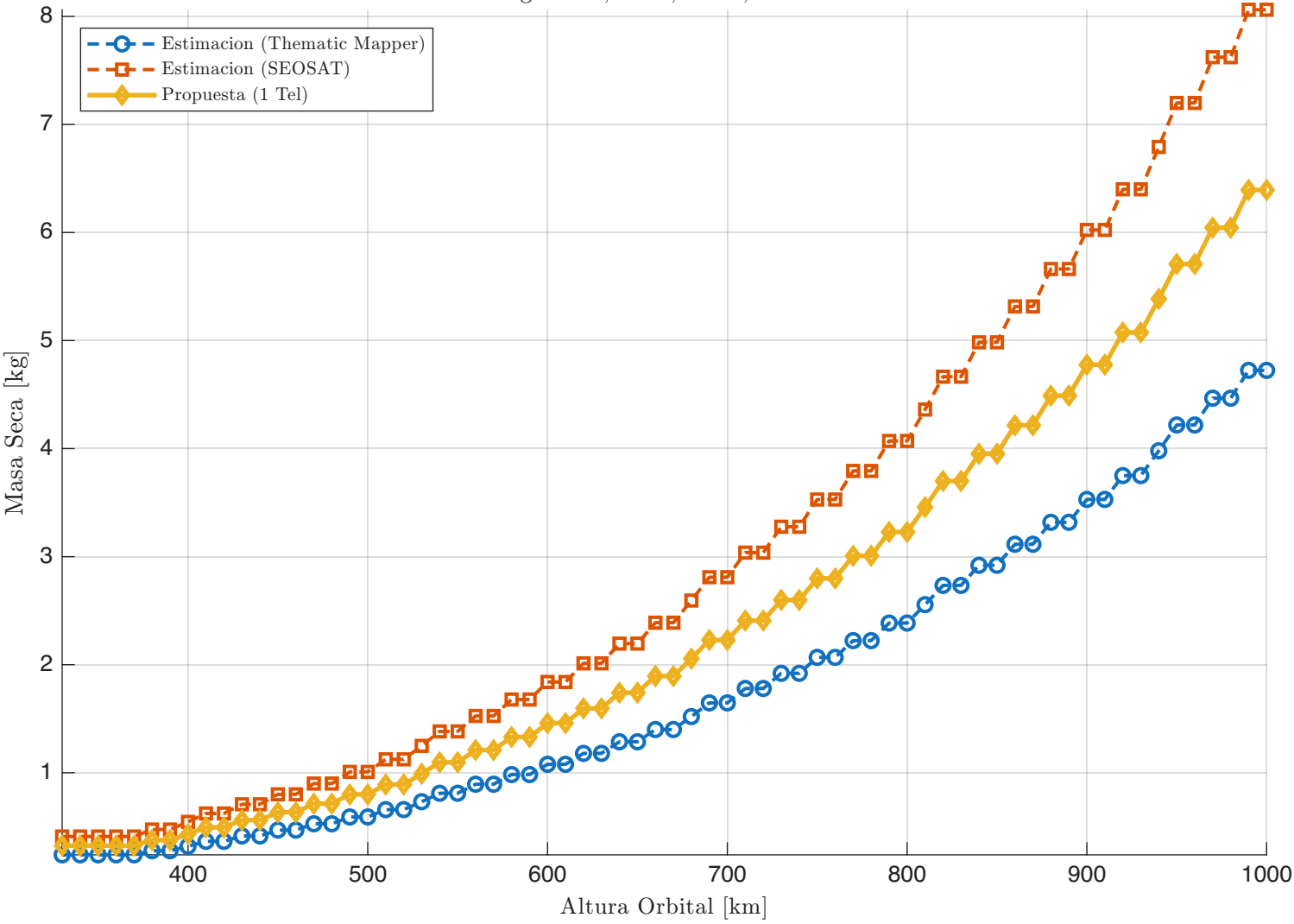
Comparativa de Masa Seca vs. Altura Config: 1 Sat, 1 Tel, Det 2, Refractivo
